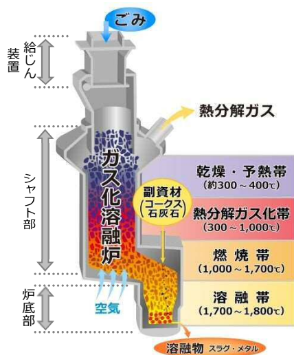
図（シャフト炉式ガス化熔融炉模式）
